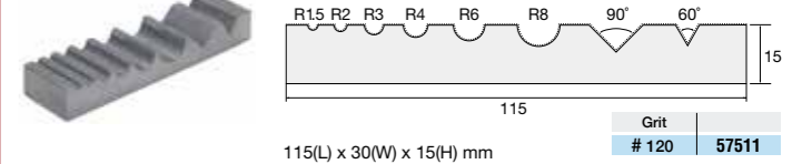
115(L) x 30(W) x 15(H) mm Grit # 120 57511
